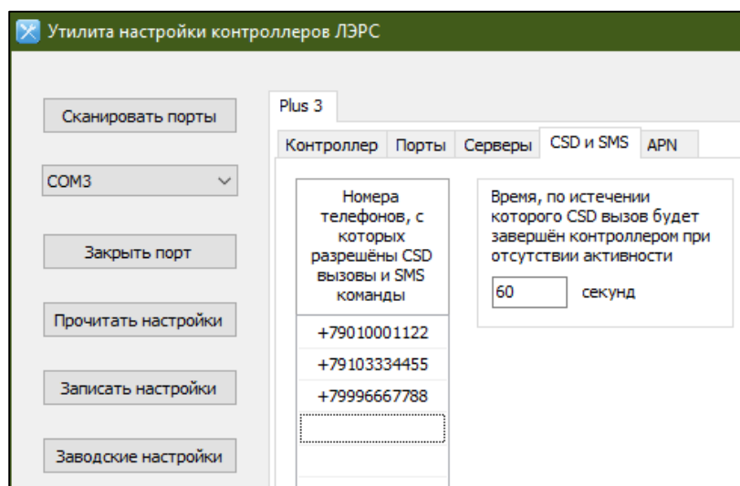
Рис. 4.5 – Утилита LersConfig, вкладка Plus3 -> CSD и SMS
